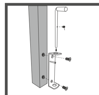
СЮРМЕ ЗА ДВУКРИЛА ВРАТА ДОЛНО
